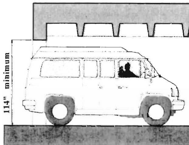
Accessible Van Space
