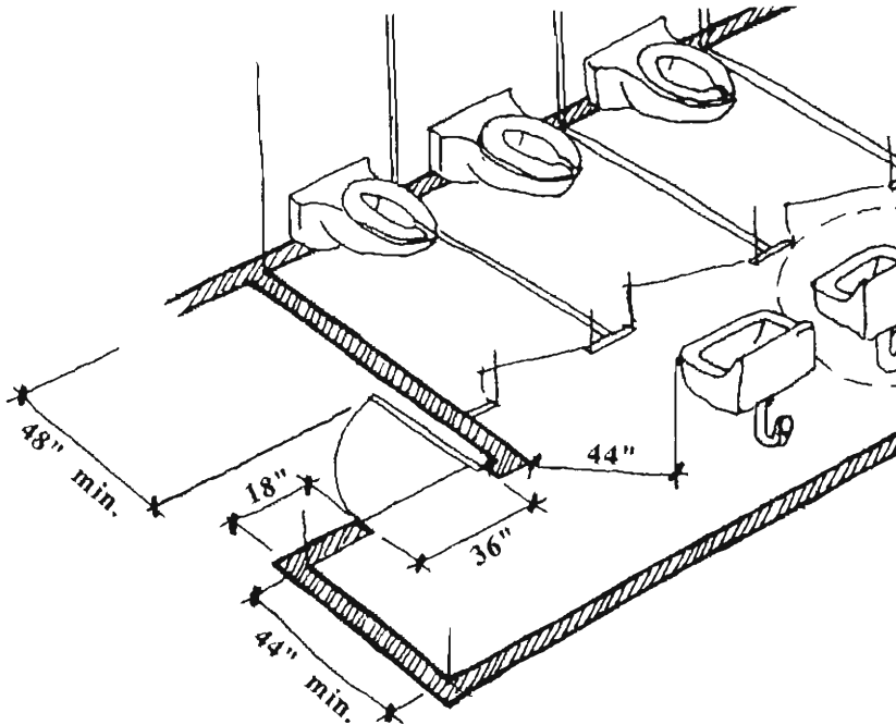
Accessible Vestibule
